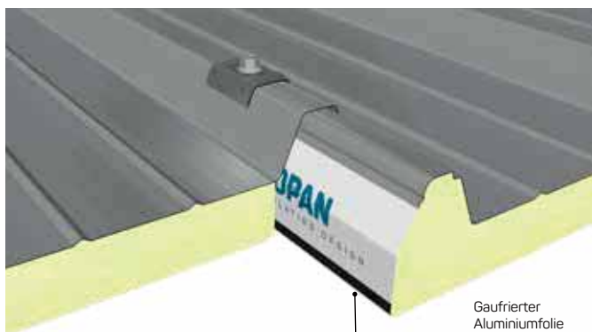
Detailansicht zu Dichtung und Befestigung
